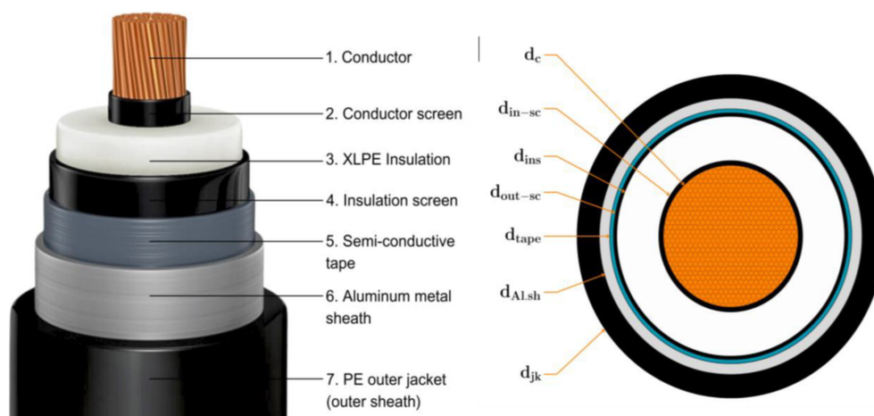
Figura 4.1: Estructura multicapa de un cable XLPE usado como referencia del objeto de estudio. Fuente: kim2025<empty citation>.
