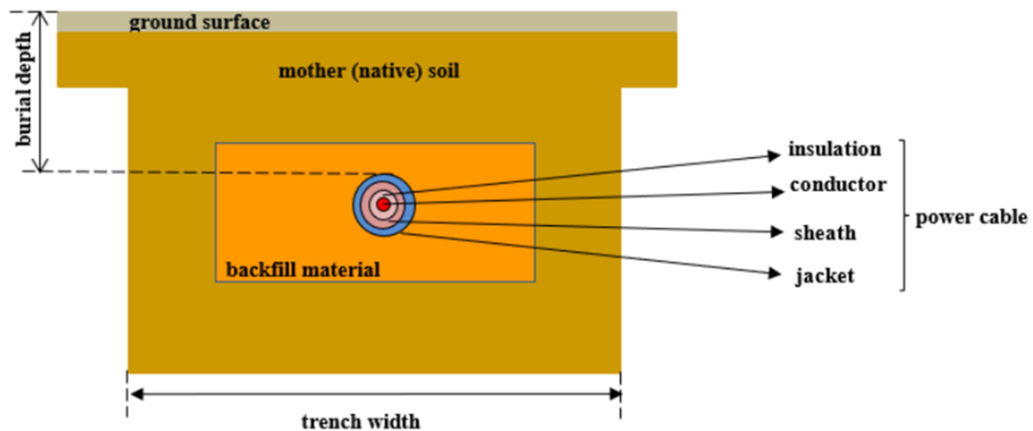
Figura 4.2: Zanja y entorno térmico del cable enterrado: relleno, suelo nativo, profundidad de instalación y capas principales del cable. Fuente: enescu2021 <empty citation>.
