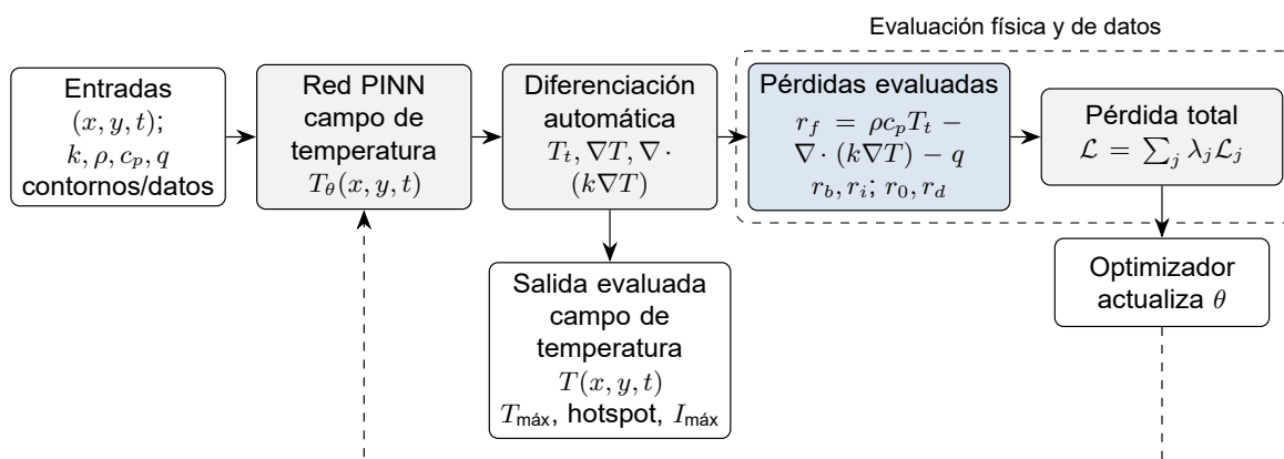
Figura 4.3: Esquema de funcionamiento de una PINN aplicada a conducción de calor. Elaboración propia a partir de raissi2019<empty citation>, lawal2022<empty citation> y pan2025<empty citation>.
